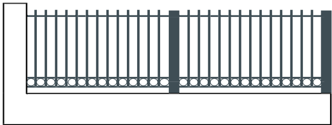
CLF 512 Clôture barreaudée avec double traverse et anneaux (festonnage en option)
