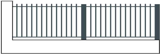
CLF 510 Clôture barreaudée (festonnage en option)
