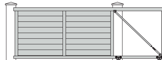
CSA 3208 : Lames droites
